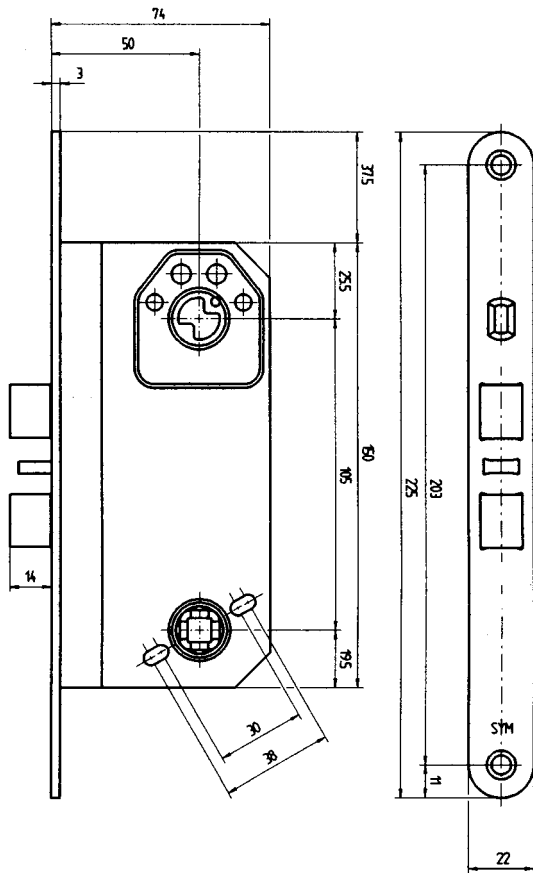
Måttskiss Modullås
