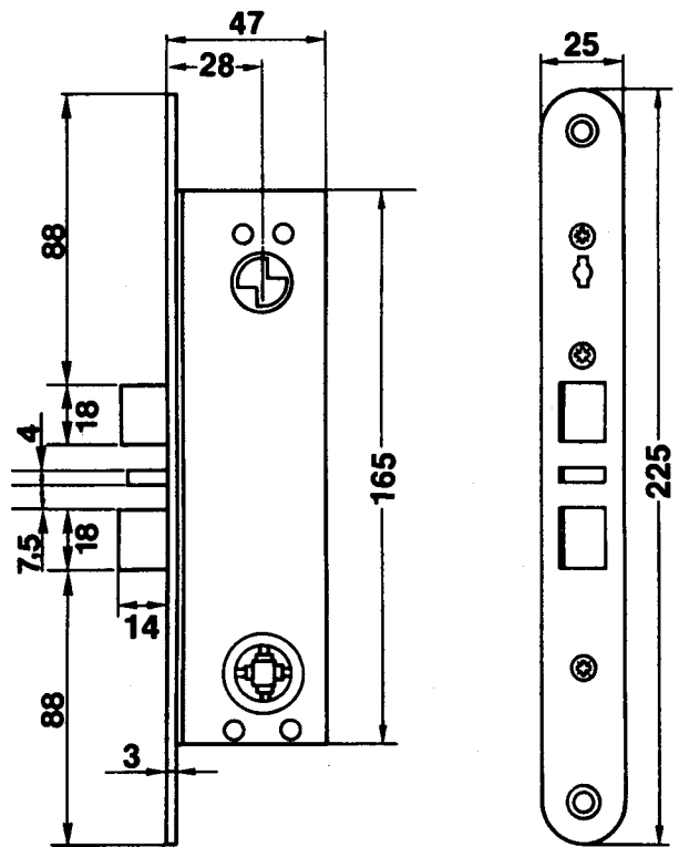
Måttskiss Smalprofilås
